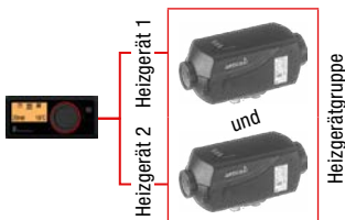
Bild 6: EasyStart Pro mit 2 Luftheizgeräten in einer Gruppe
