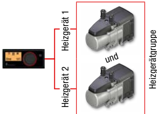
Bild 5 EasyStart Pro mit 2 Wasserheizgeräten in einer Gruppe
