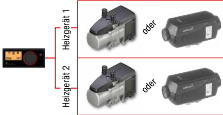
Bild 4: EasyStart Pro mit 2 separat steuerbaren Heizgeräten
